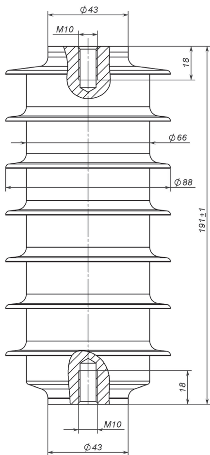
Fig. 10 PA-DH-102
