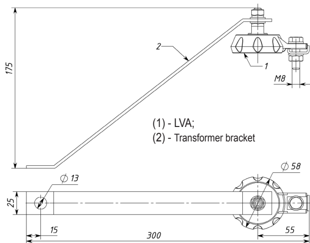
Fig. 4 PA-LVA-(MCOV)-T
