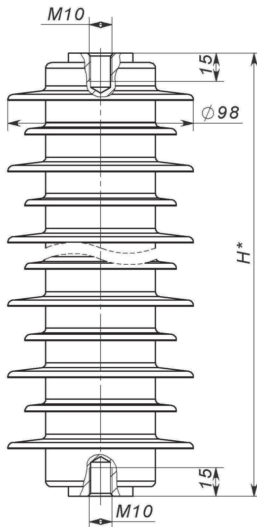
Fig. 8 PA-DM-090 ... PA-DM-098
