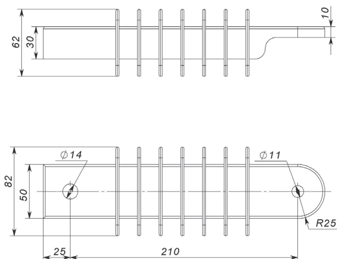
Fig. 17 Insulation bracket «I2» type. MCOV 2.55 to 29 kV
