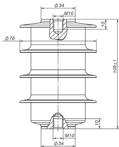
Fig. 6 PA-DM-061
