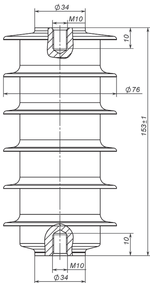
Fig. 7 PA-DM-101
