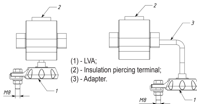
Fig. 2 PA-LVA-(MCOV)-C1
