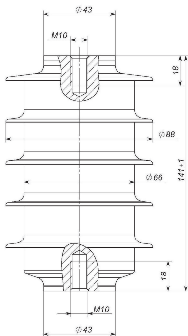
Fig. 9 PA-DH-062
