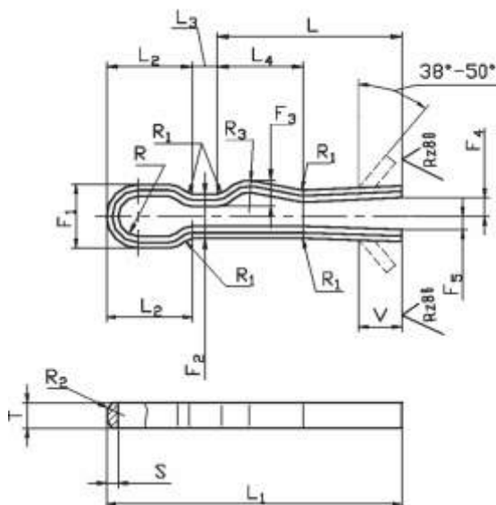
V-образные замки
