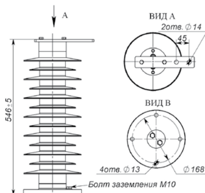
а) без изолирующего основания
