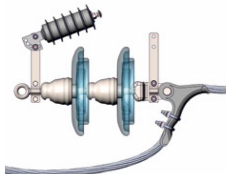
Рис.32.8 Монтаж разрядников на натяж- ную гирлянду изоляторов ПС
