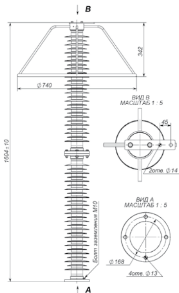
а) без изолирующего основания
