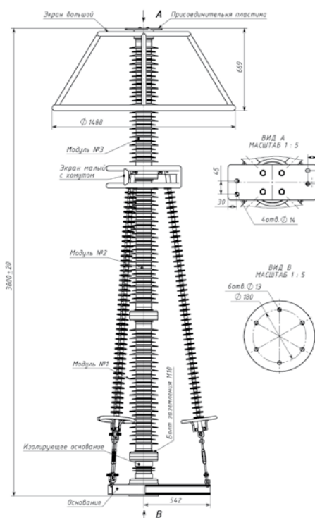
Рис.51 ОПН-330
