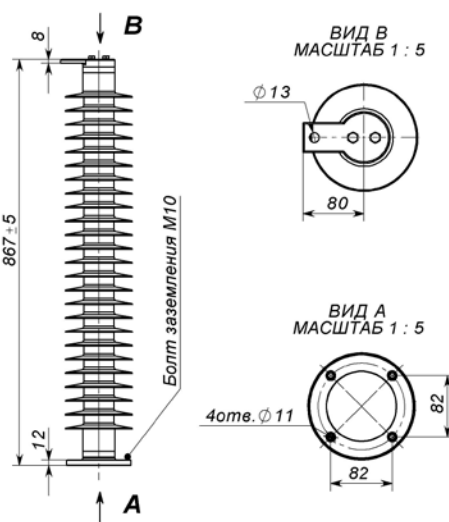
Рис. 34 ОПН-110 для нейтрали
