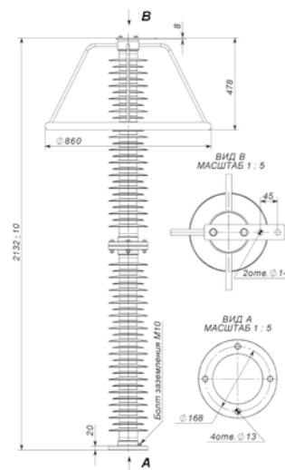
Рис. 37 ОПН-220 IV
