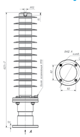
Рис. 26 ОПН-35 с Ю
