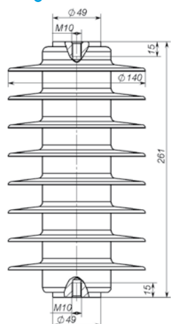
Рис. 23 ОПН-20 III
