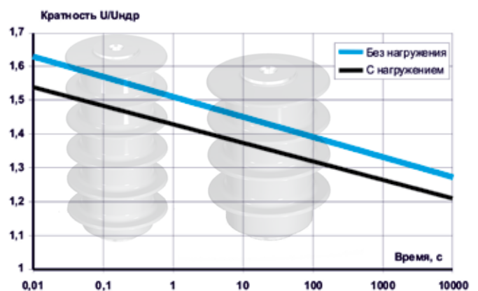
Характеристика «напряжение-время»
