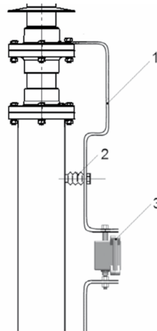
Рис.64-5 Установка ИТУС-2
