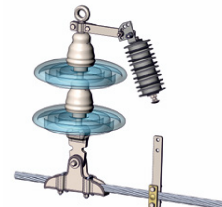
Рис.32.7 Монтаж разрядников на поддер- живающую гирлянду изоляторов ПС
