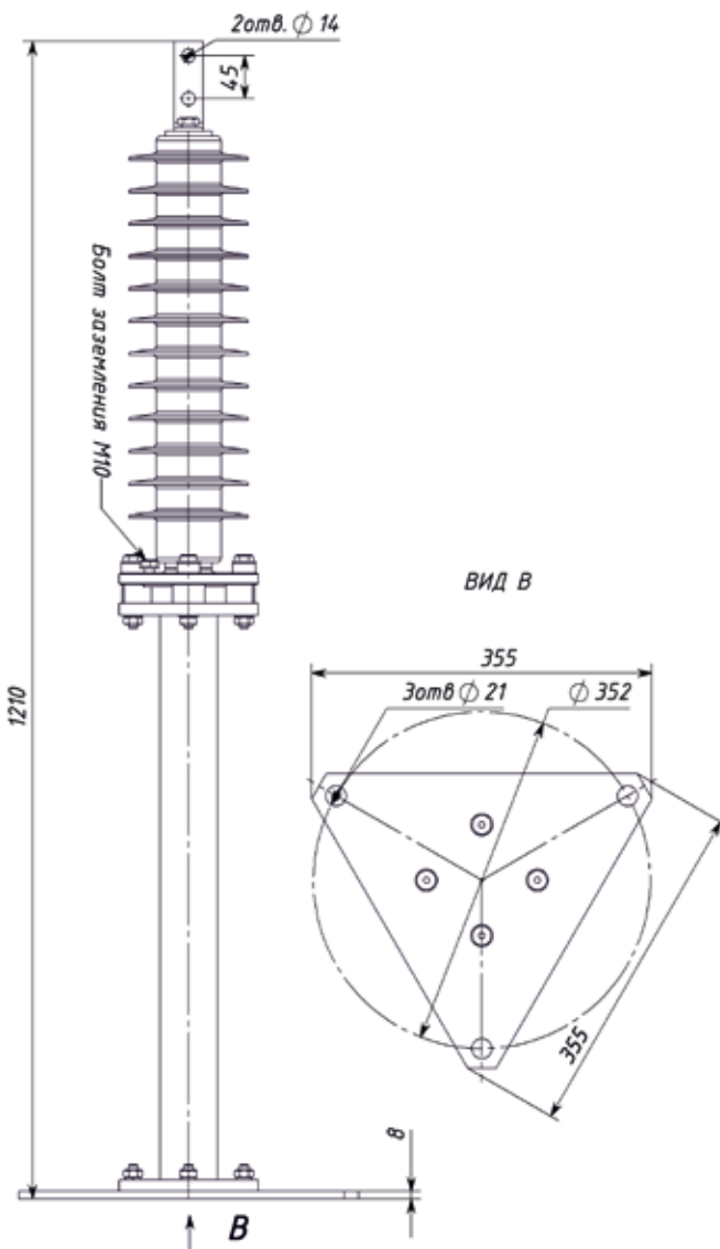
Рис.32.1 ОПН для замены РВС-35. Код исполнения «Р»
