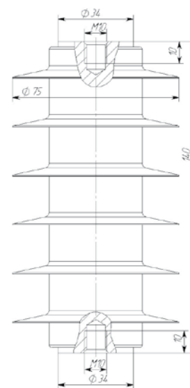
Рис. 17. ОПН-10 УХЛ2
