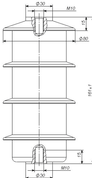
Рис. 18.5 ОПН-10 УХЛ2
