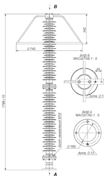
б) с изолирующим основанием
