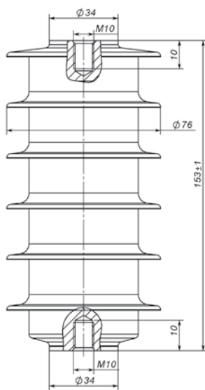
Рис. 15. ОПН-10 УХЛ1
