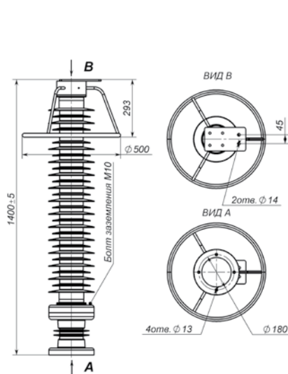
Рис.45 ОПН-110/1000 для защиты изоляции нейтрали
