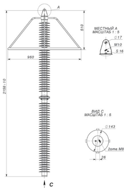
Рис.42 ОПН-220 подвесного исполнения для установки на фазные провода
