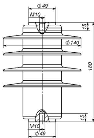
Рис. 20 ОПН-10
