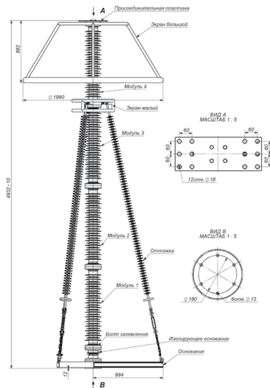
Рис.54 ОПН-500/1450(1800)
