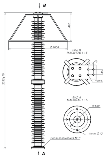
а) без изолирующего основания
