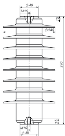
Рис. 24 ОПН-20 IV
