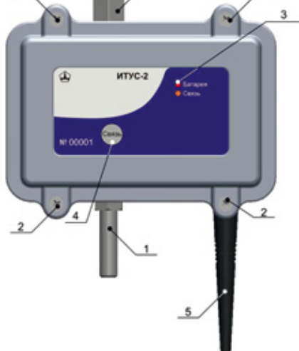
Рис.64-4 Прибор ИТУС-2
