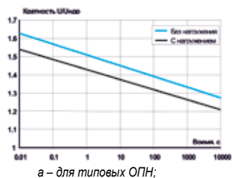
Рис. 10 Характеристика напряжения-тока
