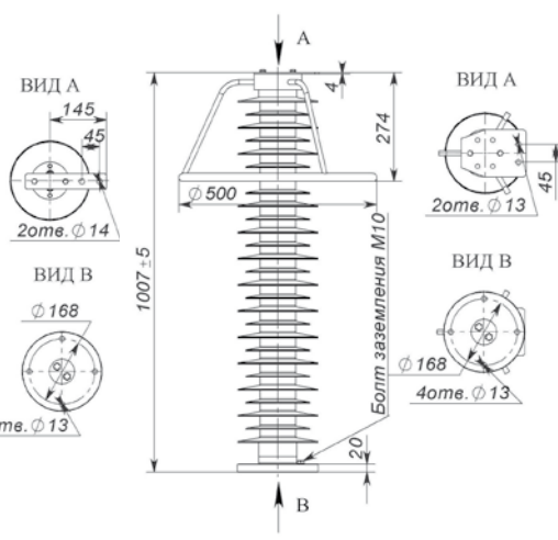
а) без изолирующего основания
