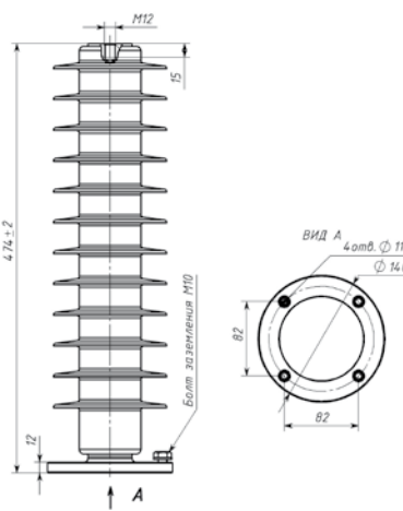
Рис. 25 ОПН-35
