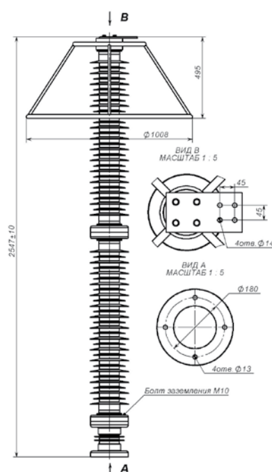
б) с изолирующим основанием
