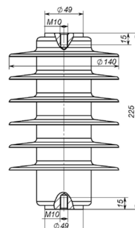
Рис. 22 ОПН-15 IV
