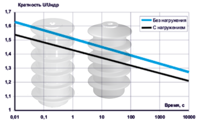
Характеристика «напряжение-время»
