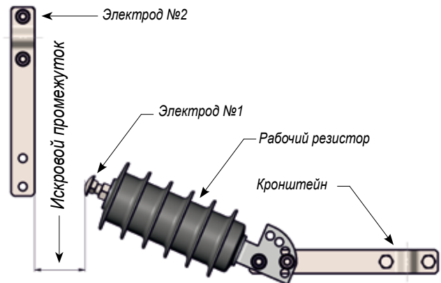
Рис. 32.2 Разрядник вентильный линейный (РВЛ) классов напряжения 6 ÷ 20 кВ
