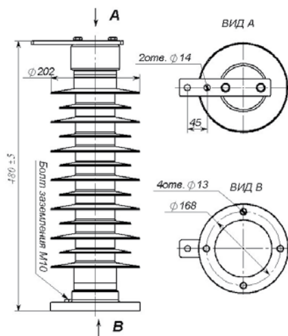
Рис.43 ОПН 6-15 кВ для генераторных РУ
