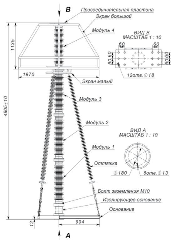
Рис.55 ОПН-500/2100(3200)
