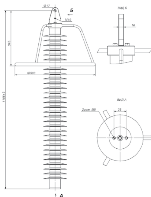
Рис.41 ОПН-110 подвесного исполнения для установки на фазные провода
