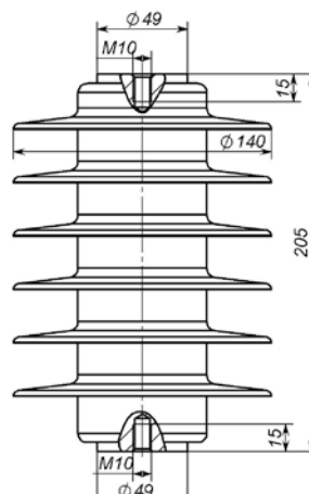
Рис. 21 ОПН-15 III
