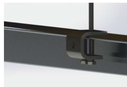
Крепление устройства на горизонтальную полку траверсы
