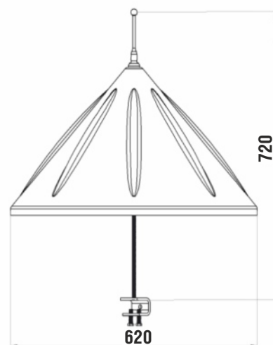
Габаритные размеры ПЗУ-BL-PA 720
