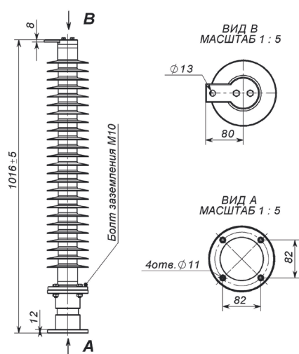
Рис.38 ОПН-110 для защиты изоляции нейтрали
