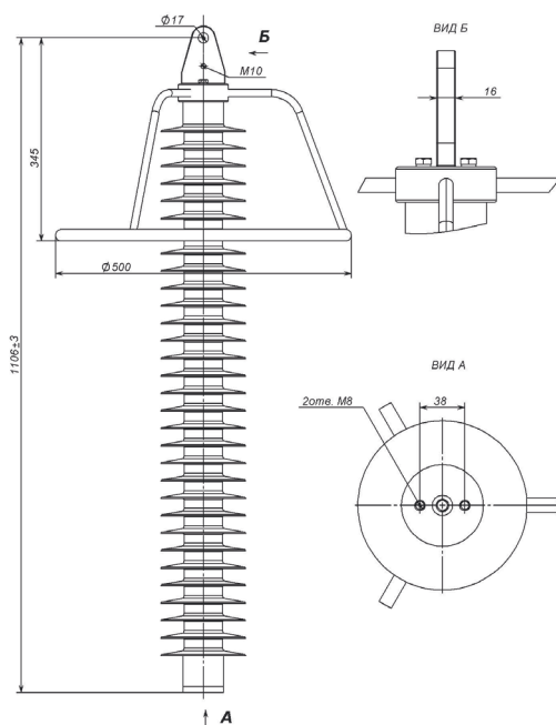
Рис.41 ОПН-110 подвешного исполнения для установки на фазные провода
