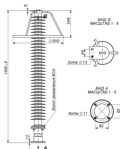
Рис.40 ОПН-110 IV с усиленной изоляцией для установки под фазное напряжение
