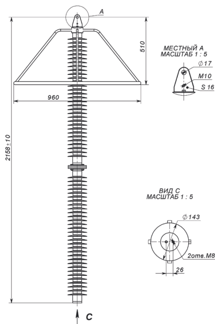
Рис.42 ОПН-220 подвешного исполнения для установки на фазные провода
