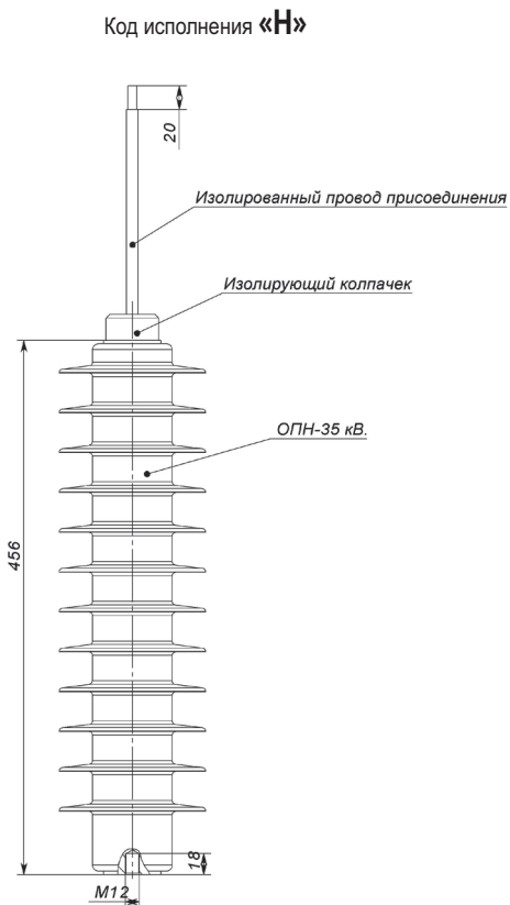
Рис.30 ОПН с изолированным подключением
