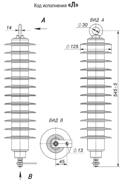
Рис.29 ОПН подвешного исполнения с отделителем
