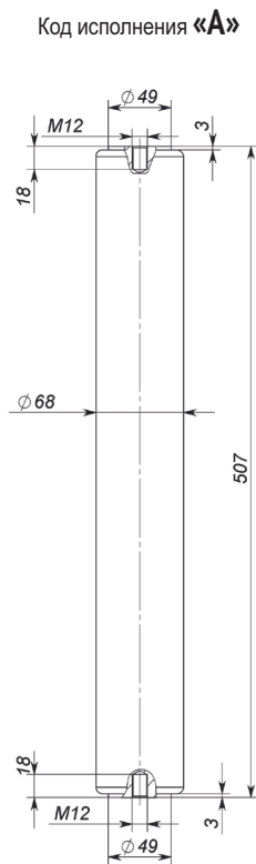
Рис.31 ОПН для установки в ячейки кабельных присоединений
