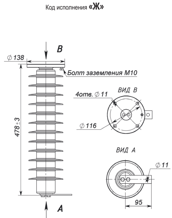
Рис.29 ОПН подвешного исполнения с отделителем
