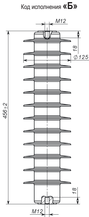
Рис.27 ОПН без основания
