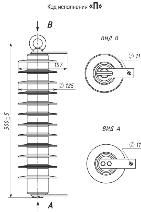
Рис.28 ОПН подвешного исполнения
